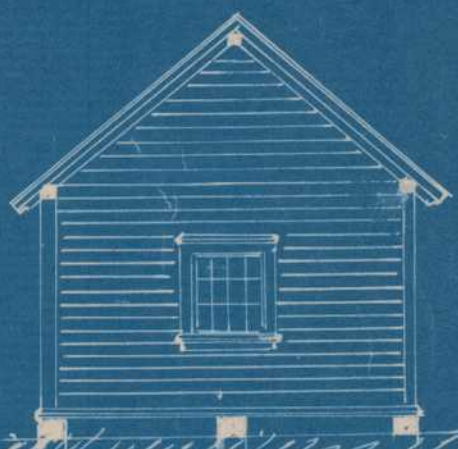
GAVL-FASADE
