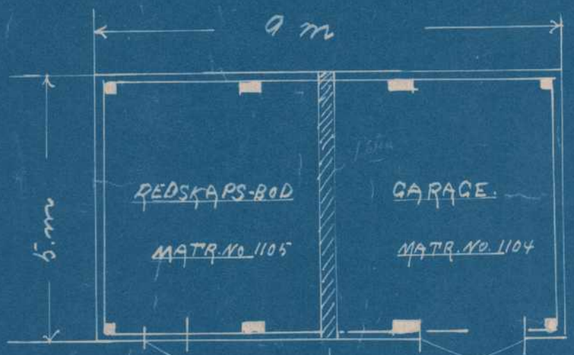
GRUNDPLAN
