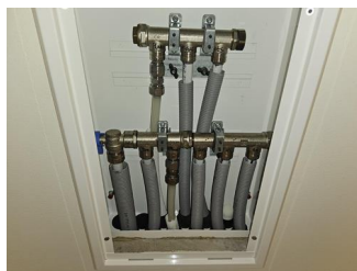
Fordelerskap og fordelerstammer - Fordelerskap i himling på bad
