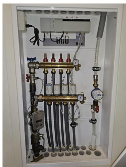
Vannbåren varme (radiatorer, vannbåren gulvvarme, o.l.) - Fordeling vannbåren gulvvarme.
