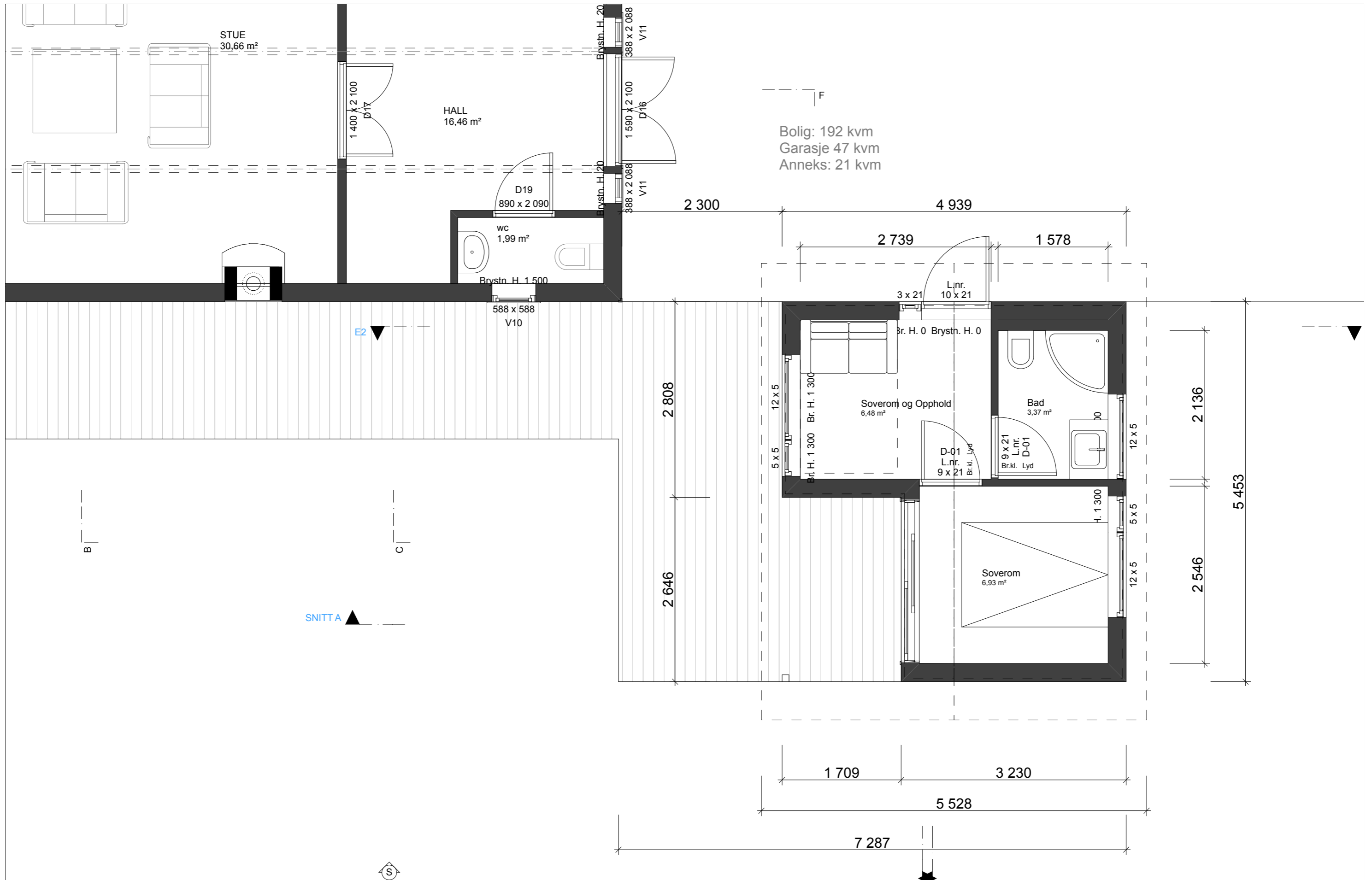
1. HOVEDPLAN
