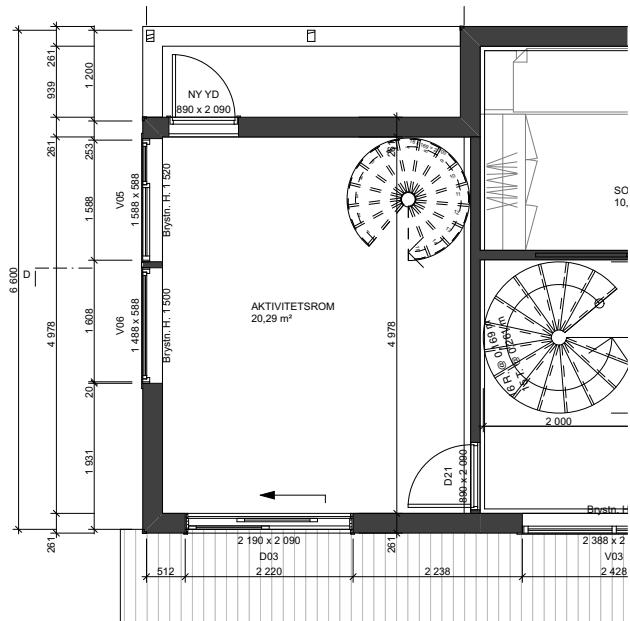
1. HOVEDPLAN 1:100
