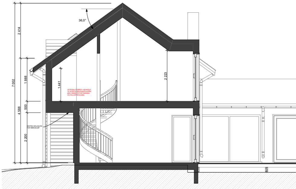
SNITT A-A 1:100
