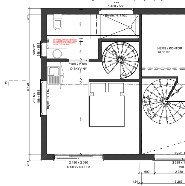
1. PLAN 2.ETG 1:100
