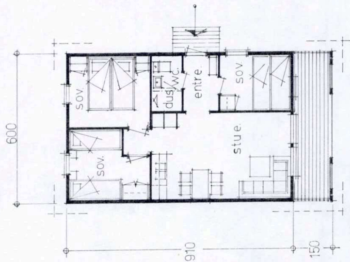
PLANLØSNING
